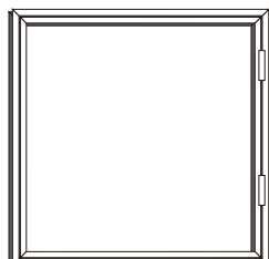
Рама открывающаяся одностворчатая из профильной трубы: 20x20x2 - РО01 25x25x2 - РО02
