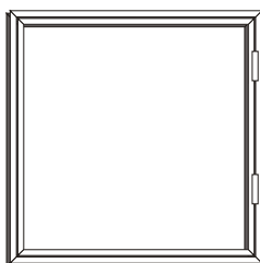
Рама открывающаяся одностворчатая из профильной трубы: 20x20x2 - РО01 25x25x2 - РО02
