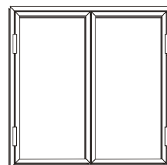
Рама открывающаяся двустворчатая из профильной трубы: 20x20x2 - РД01 25x25x2 - РД02
