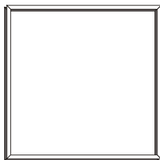
Рама глухая из профильной трубы: 20x20x2 - РП01 из уголка: 25x25x4 - РУ01 32x32x4 - РУ02
