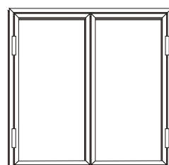
Рама открывающаяся двухстворчатая из профильной трубы: 20x20x2 - РД01 25x25x2 - РД02
